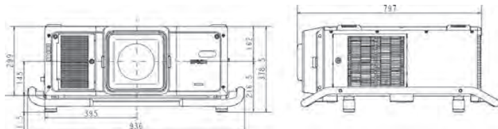
■外形寸法 (単位: mm)
