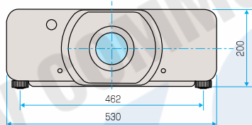
■外形寸法 単位：mm
